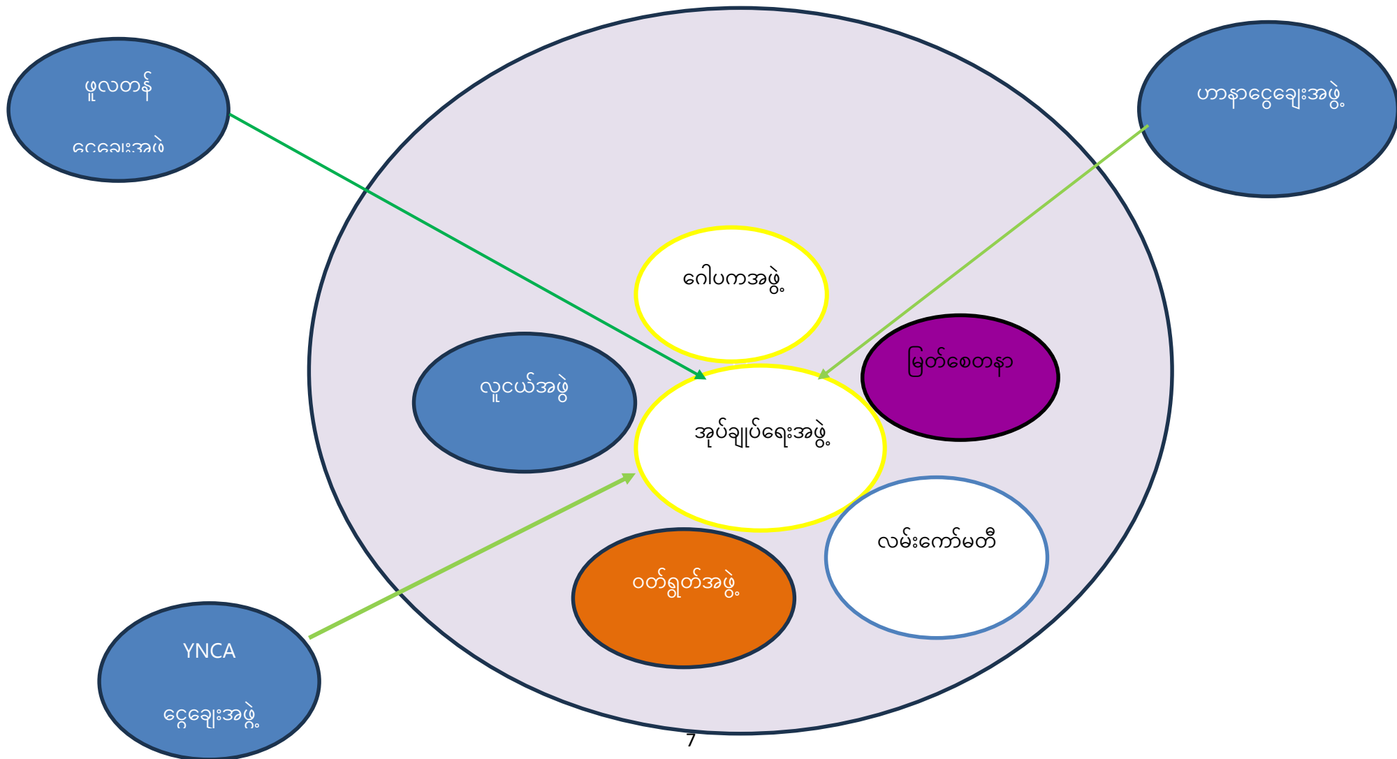
Venn Diagram
